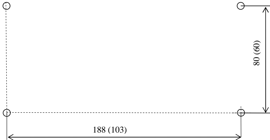
Рисунок 9.6. Разметка крепления корпуса УПВК-1У исп.2 и УППВК- значения в скобках.
