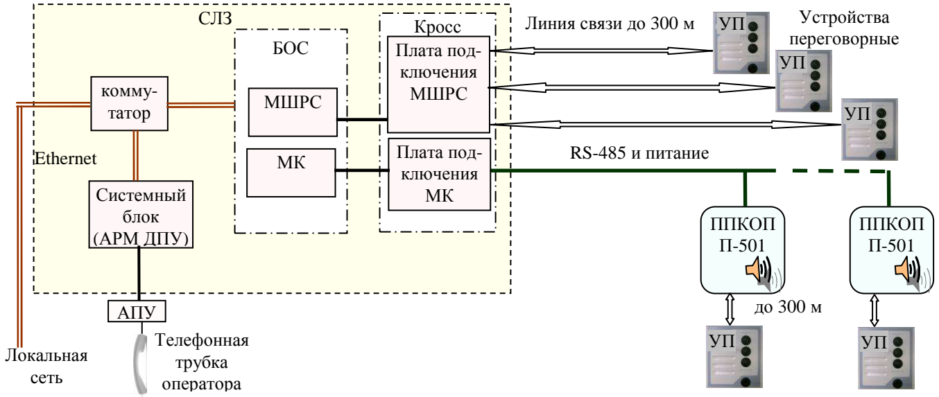
Рисунок 11.1 Структурная схема системы речевой связи
