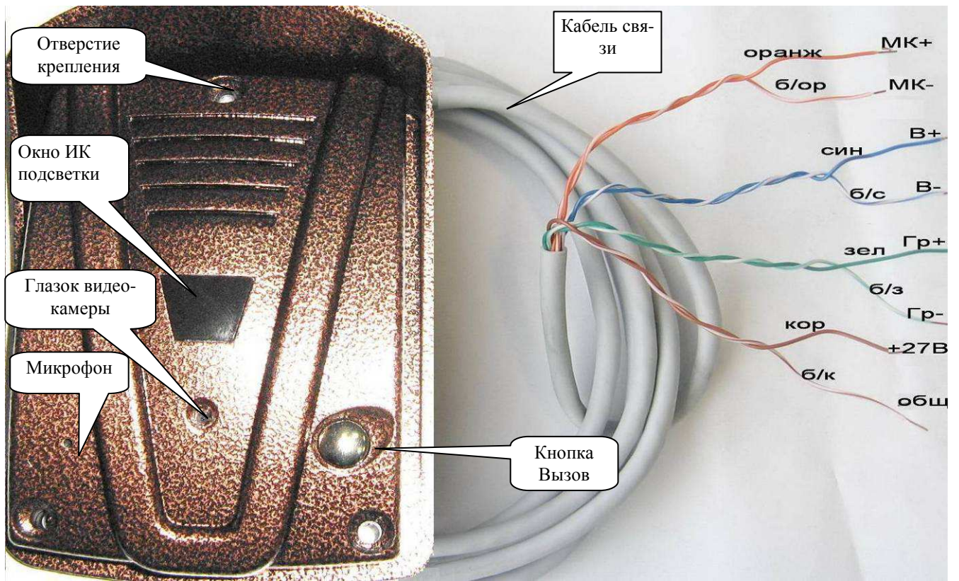
Рисунок 11.11 УЭВ исп.2 вид спереди
