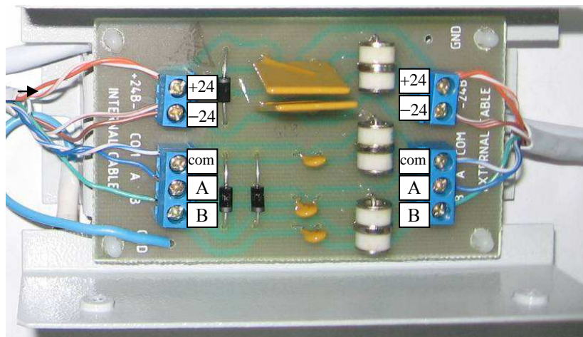
Рисунок 10.15 Подсоединение к УВЗ
