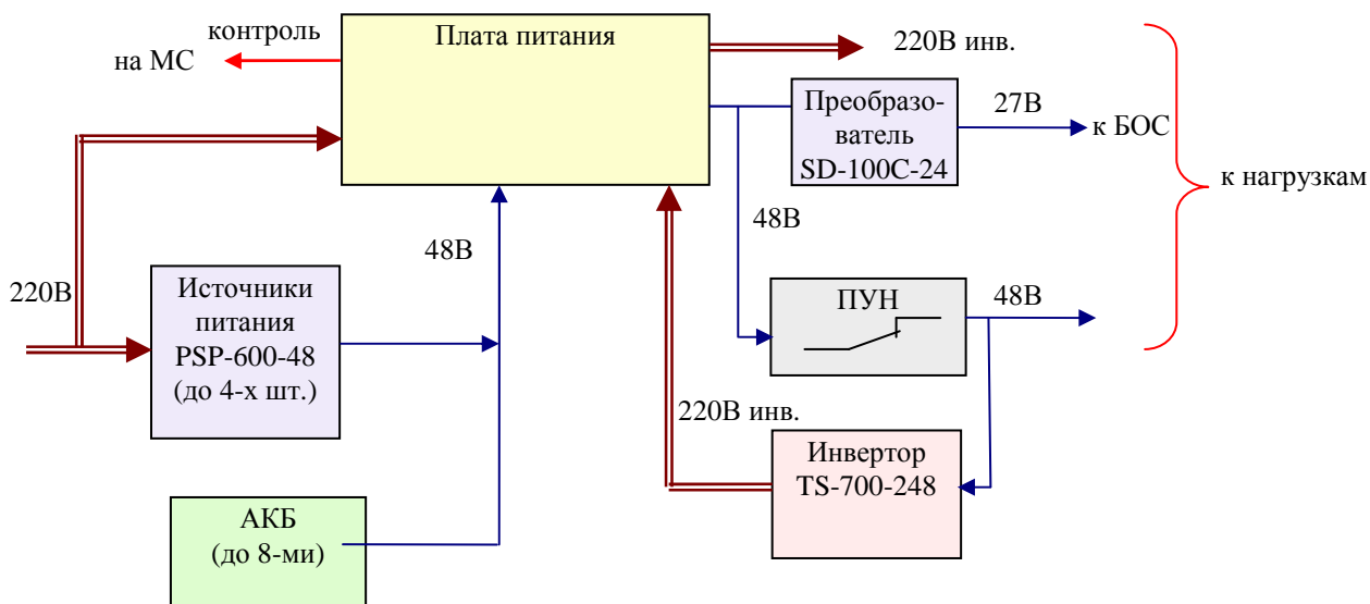
Рисунок 5.12. Структурная схема БП СЛЗ.
