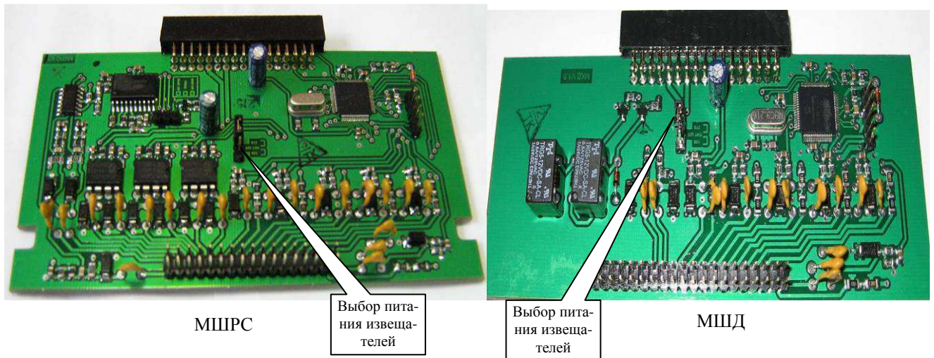
Рисунок 10.2. Установка напряжения питания извещателей в МШРС и МШД
