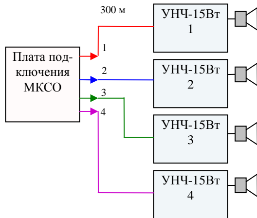
Рисунок 12.3 Параллельное подключение УНЧ-15Вт
