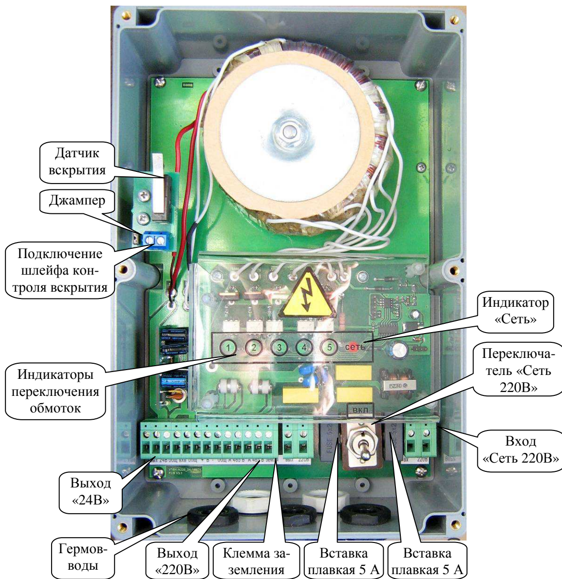
Рисунок 9.15 УПК-А220 со снятой крышкой
