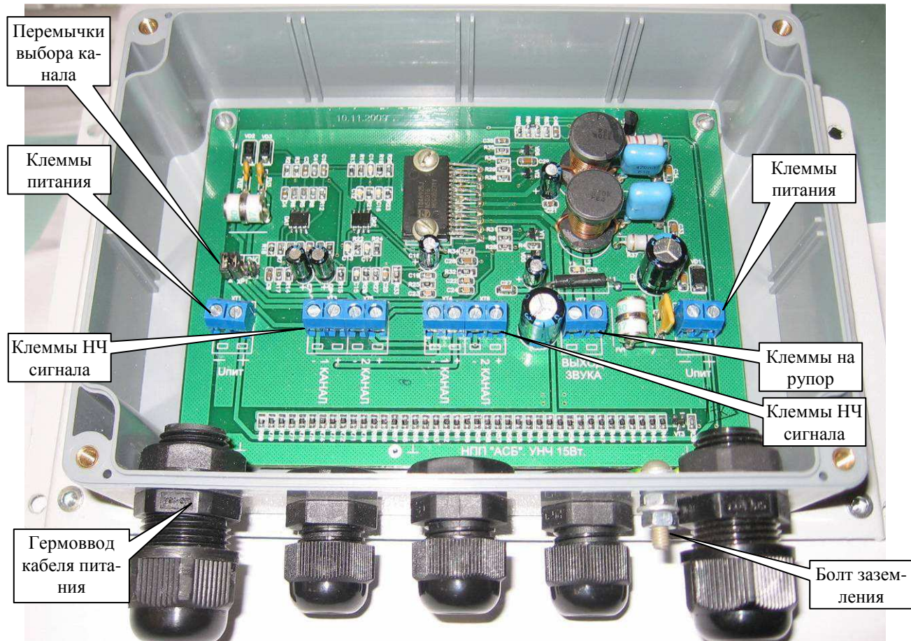
Рисунок 12.5 Вид УНЧ-15Вт со снятой крышкой
