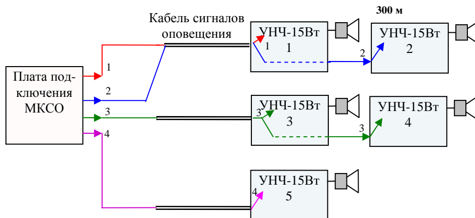
Рисунок 12.4. Последовательно-параллельное подключение УНЧ-15Вт
