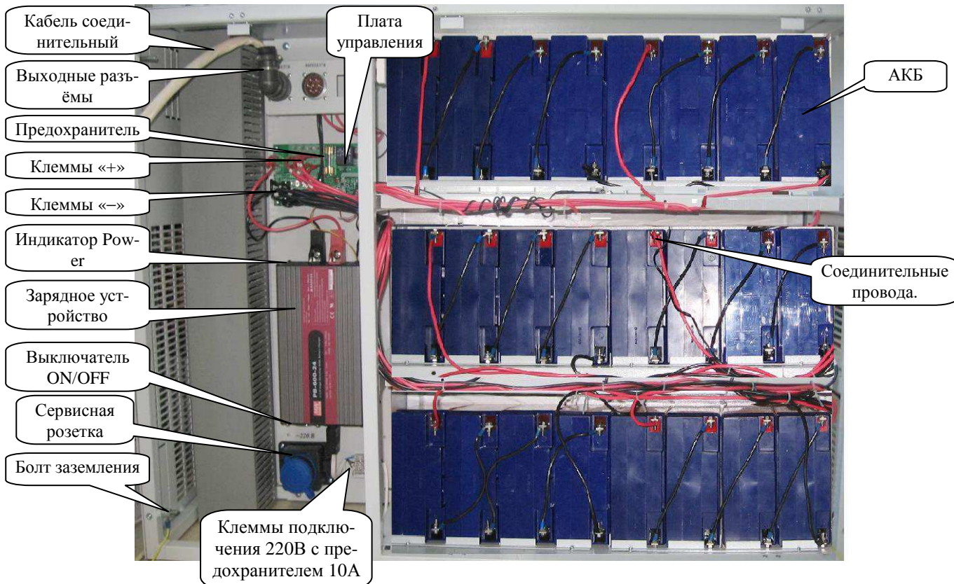
Рисунок 16.2 Вид БРП-48В-108Ач со снятыми дверцами
