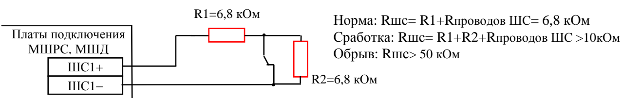
г) Подключение двух резисторов к размыкающему контакту с разделением «Обрыв» и «Тревога»
