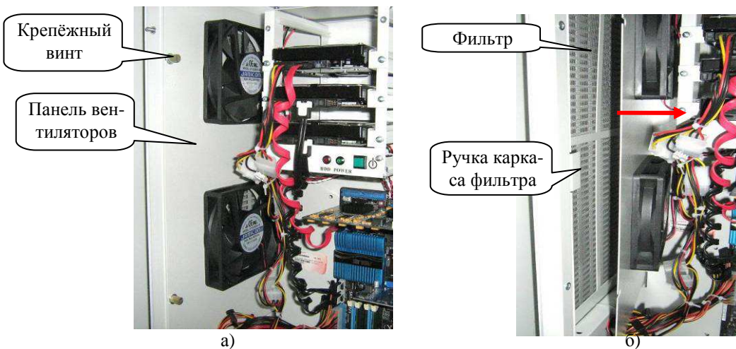
Рисунок 19.1 Снятие фильтра вентилятора
