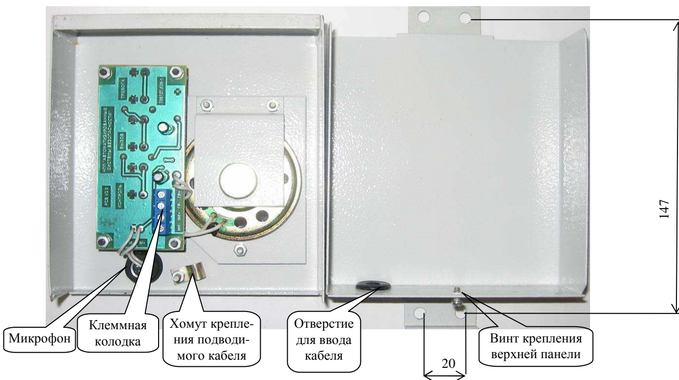
Рисунок 11.4 УП-1
