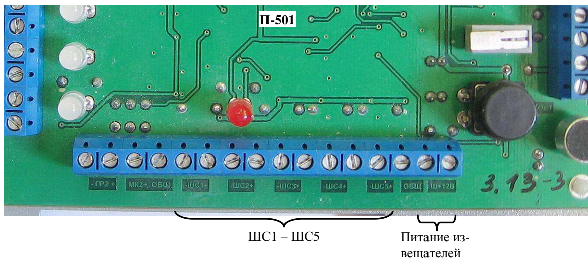
Рисунок 10.13. Клеммы П-501 для подсоединения извещателей
