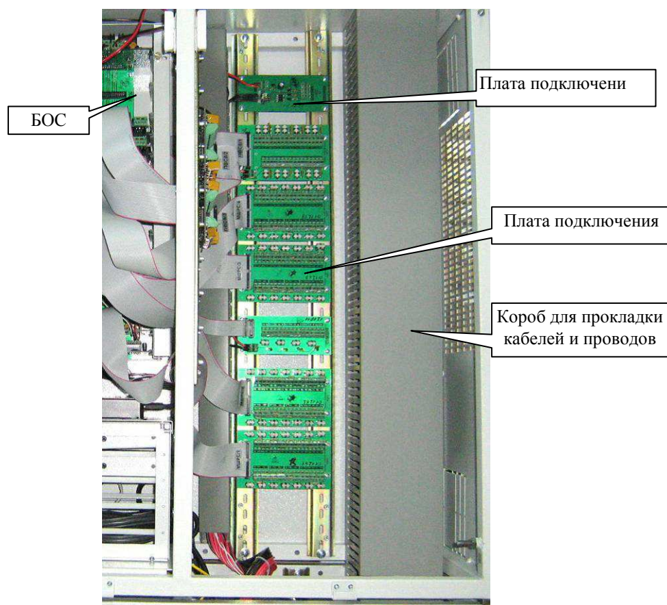
Рисунок 5.2. Кросс-панель сервера.
