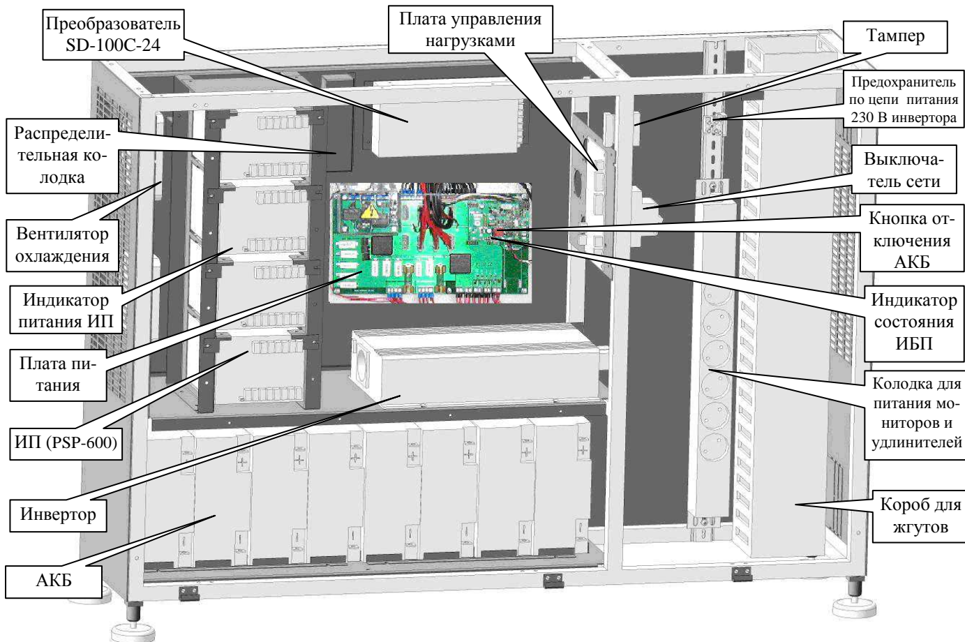
Рисунок 5.11 Вид БП со снятыми передними дверцами.
