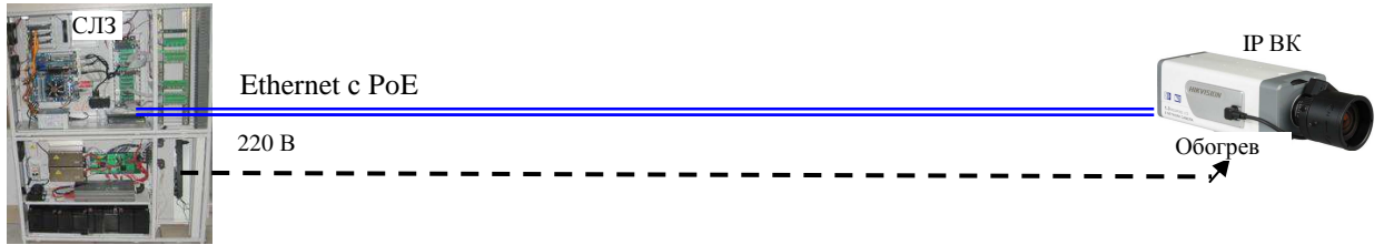
б) подключение IP ВК с питанием по витой паре в сети Ethernet.
