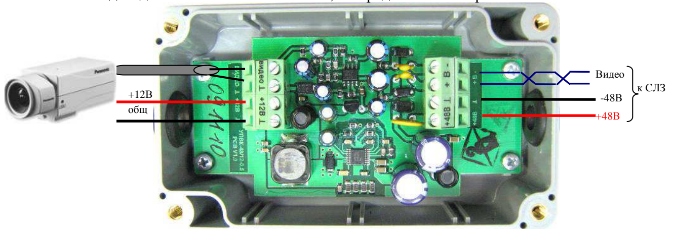
Рисунок 9.8 Подключение кабелей к УПВК-0,3П исп.2
