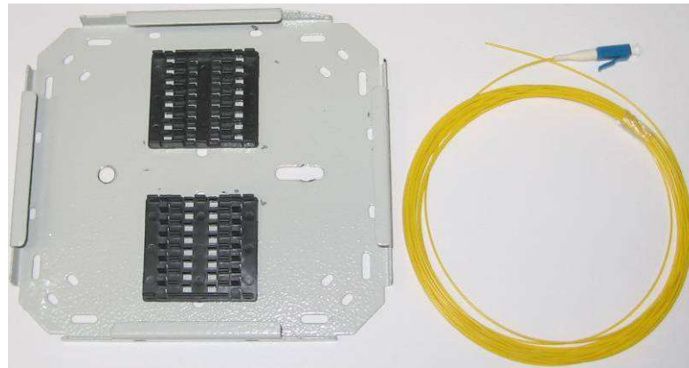
Рисунок 7.13. Сплайс-пластина и пигтейл.
