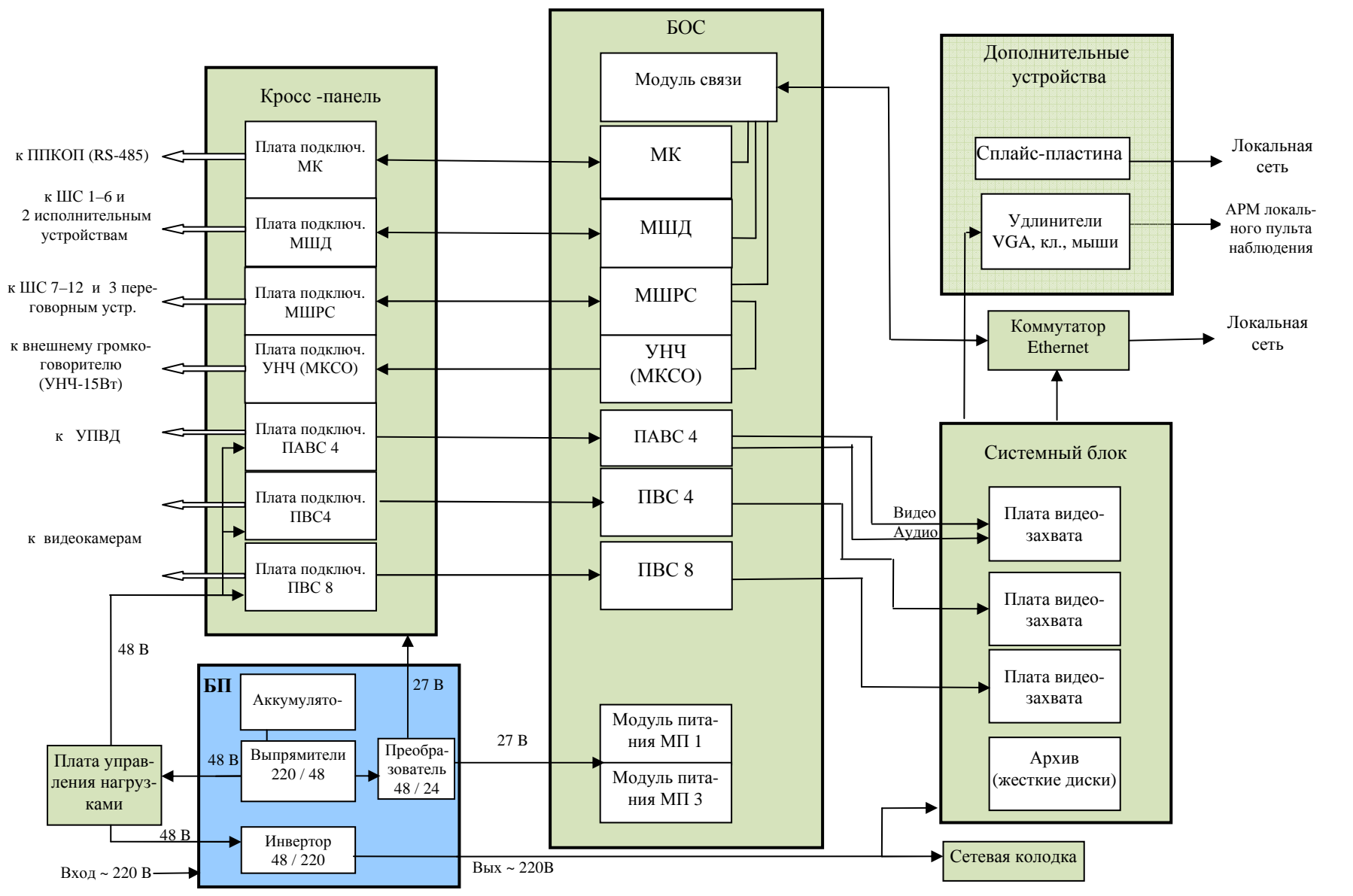
Рисунок 5.1. Структурная схема СЛЗ
