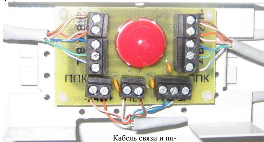
Рисунок 10.16 Подсоединение к УПЗ
