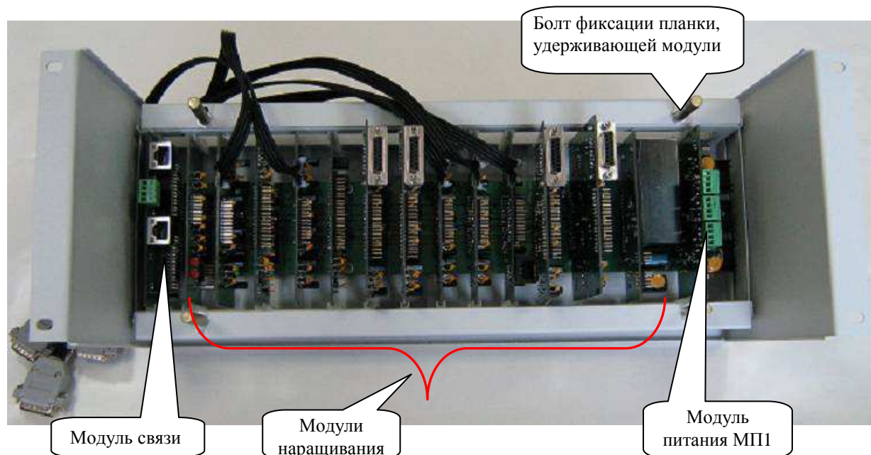
Рисунок 5.3 . Внешний вид блока обработки сигналов с установленными модулями.
