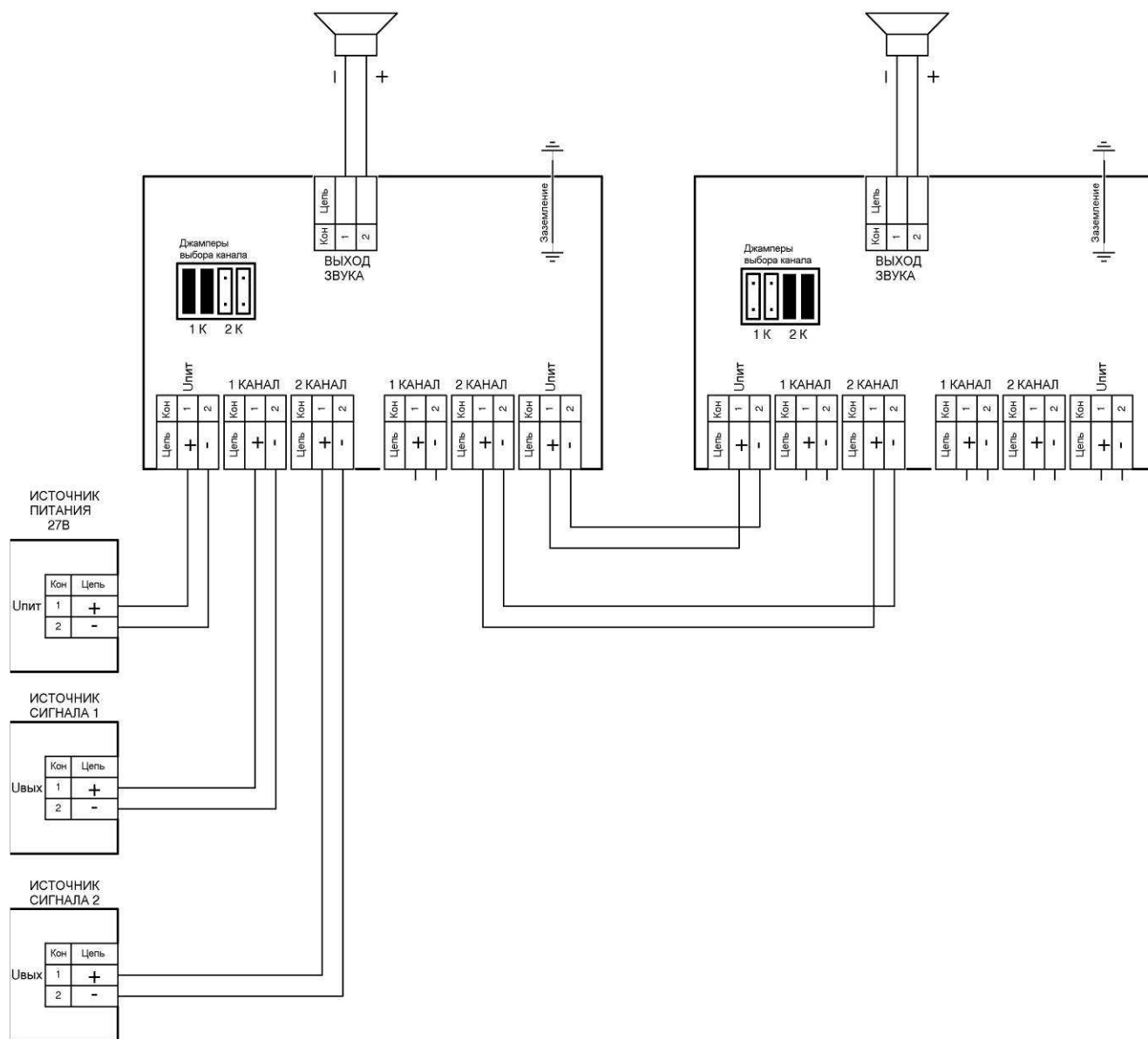
Рисунок 12.8 Пример работы двух УНЧ-15Вт от двух сигналов оповещения
