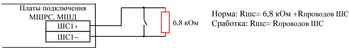
а) Параллельное подключение резистора без разделения «КЗ» и «Тревога»
