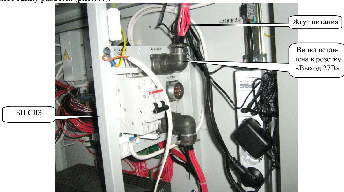
Рисунок 7.4. Подключение жгута питания
