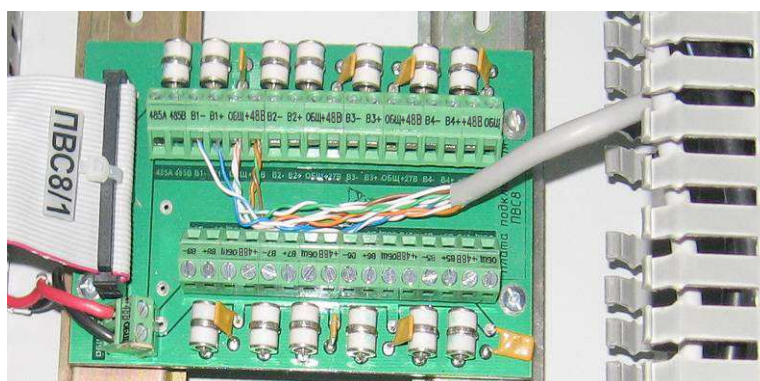
Рисунок 9.11. Подсоединение линии связи к плате подключения ПВС8 (8 каналов).
