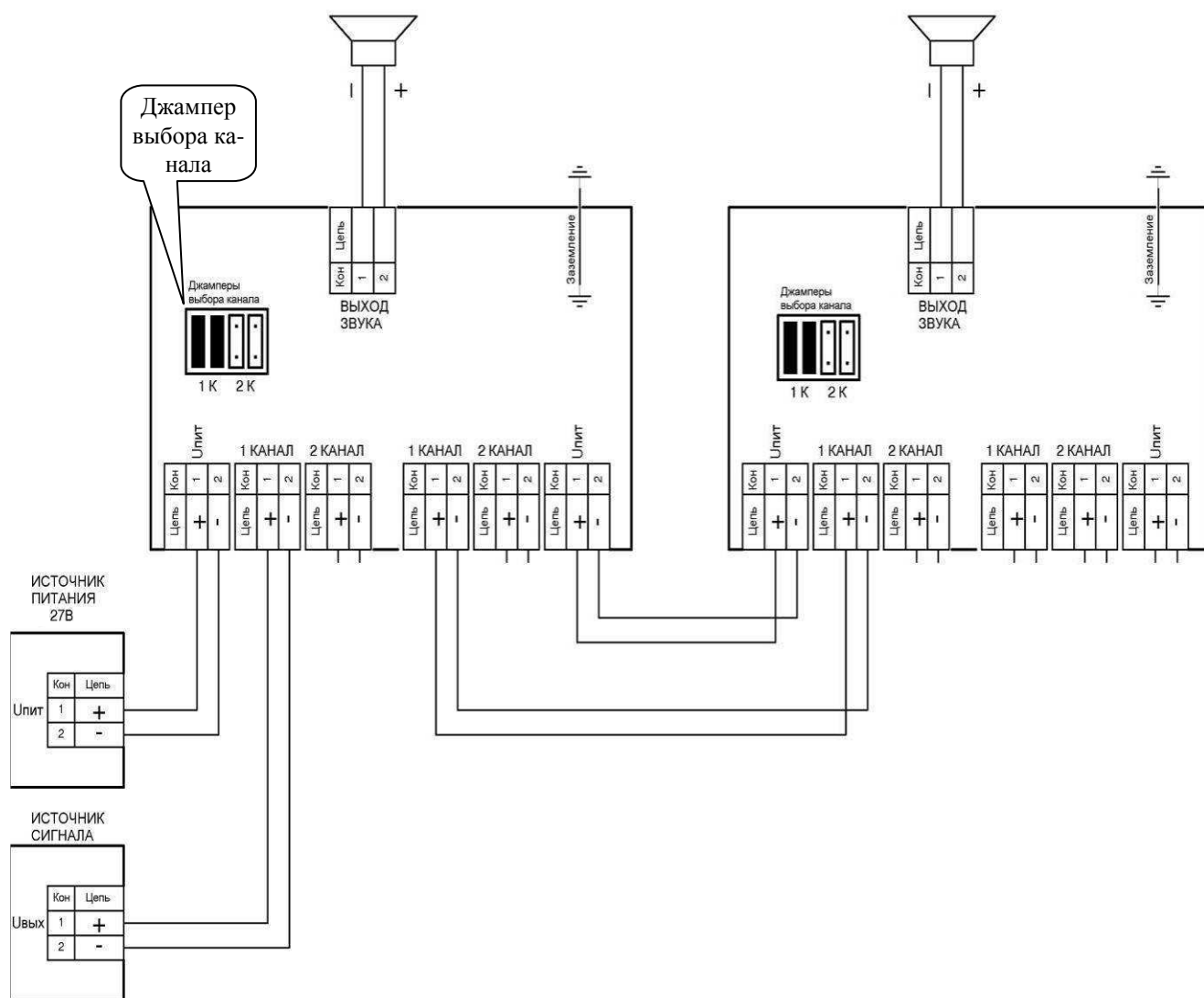
Рисунок 12.7 Пример работы двух УНЧ-15Вт от одного сигнала оповещения
