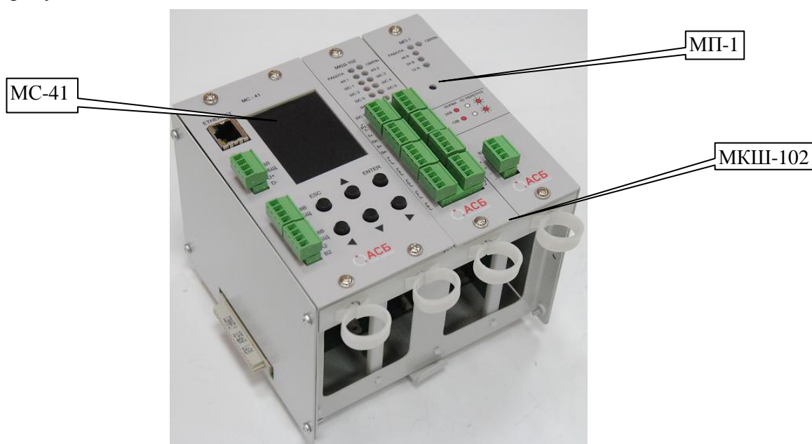
Рисунок 1 - Прибор МС-41 в составе корзины АК-4D
