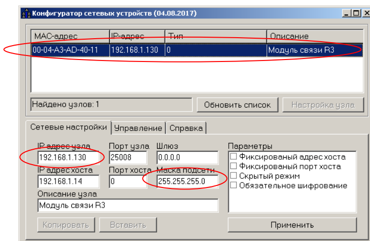
Рисунок 5 - Интерфейс утилиты npr.exe
