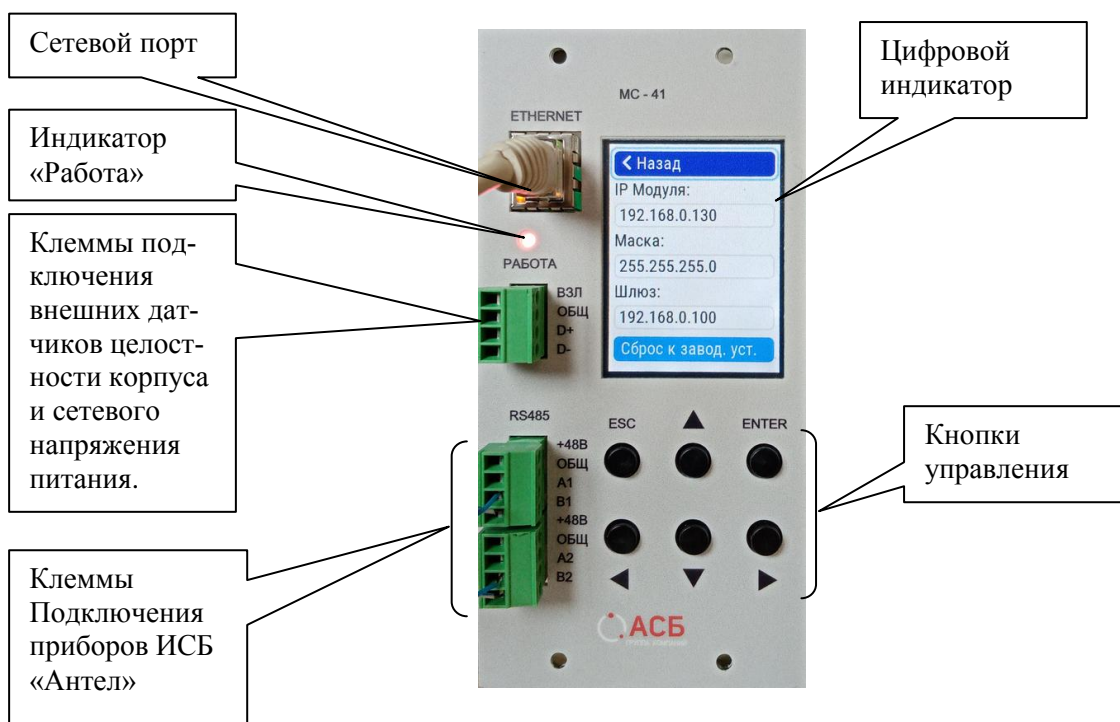
Рисунок 3 - Передняя панель MC – 41
