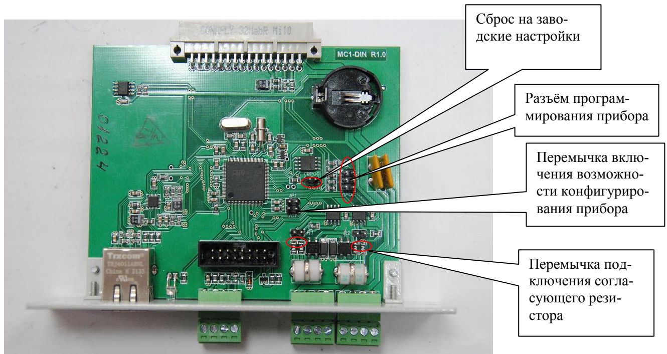
Рисунок 4 - Печатная плата МС-41
