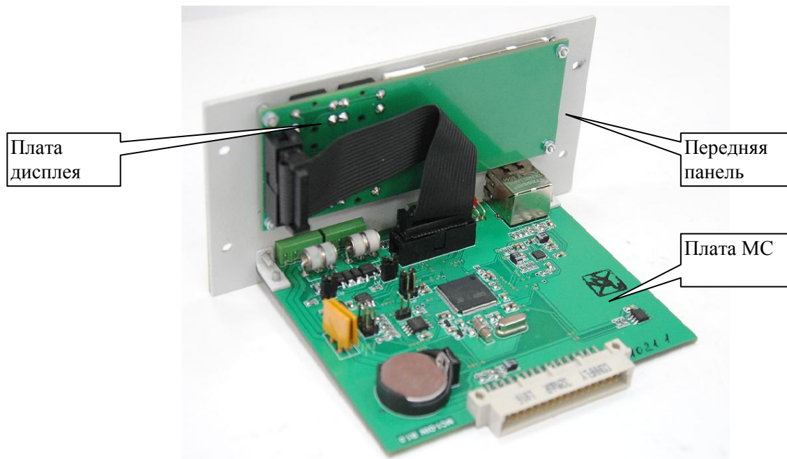
Рисунок 2 - Общий вид прибора
