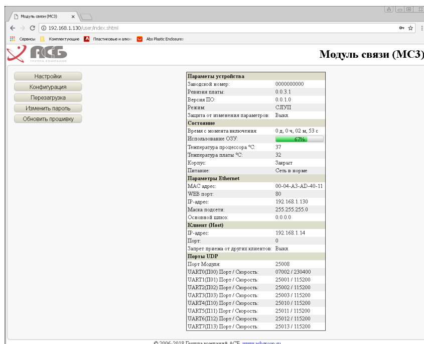
Рисунок 6 - Главная страница веб-интерфейса МС
