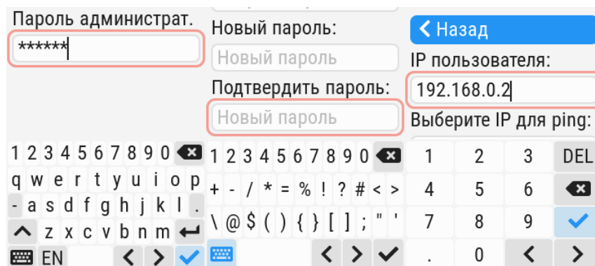
Рисунок 9 - Экранная клавиатура
